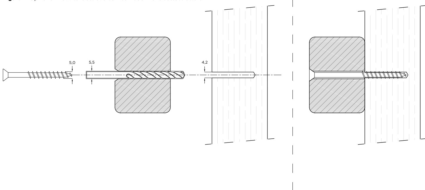
Figura 2. Opzione 2 : avvitare attraverso il bamboo in una sottostruttura
