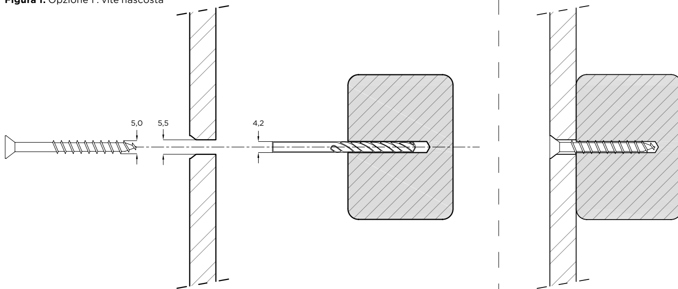
Figura 1. Opzione 1: vite nascosta
